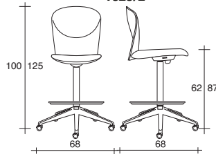
VULCAN 1325/Z
