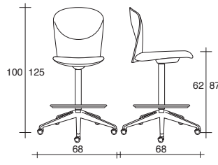
VULCAN 1325/Z
