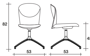
VULCAN 1295/Z
