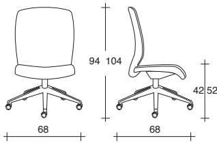
DIESIS PLUS 271/M
