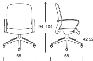
DIESIS PLUS 272/M
