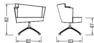
ELIPSE EL 1RX
