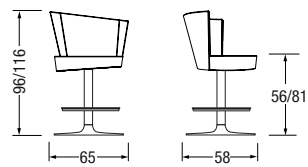
ELIPSE EL 10/HG
