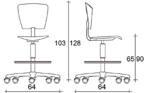
VEKTA 103/H
