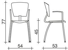
VEKTA 101
