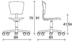
VEKTA 103
