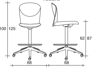
VULCAN 1325/Z
