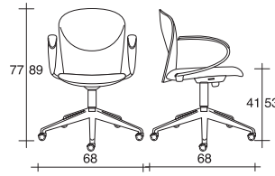
VULCAN 1316/Z
