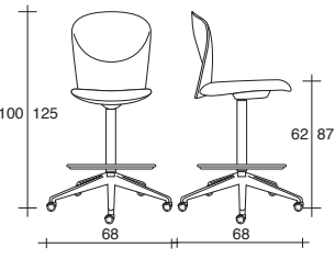
VULCAN 1325/Z
