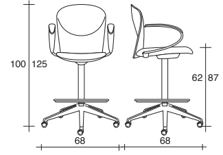
VULCAN 1330/Z
