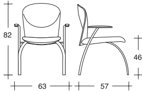
VULCAN 1275/ZTdx
