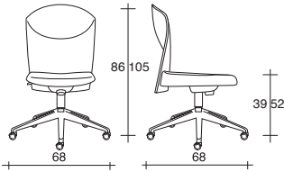
VULCAN 1405/Z
