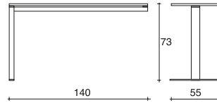
KOMPACT 893/C
