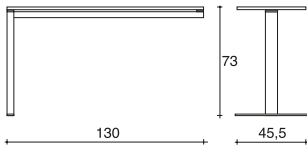
KOMPACT 888/C
