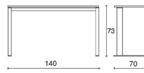
KOMPACT 896
