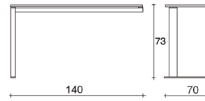
KOMPACT 896/C
