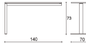
KOMPACT 897/C
